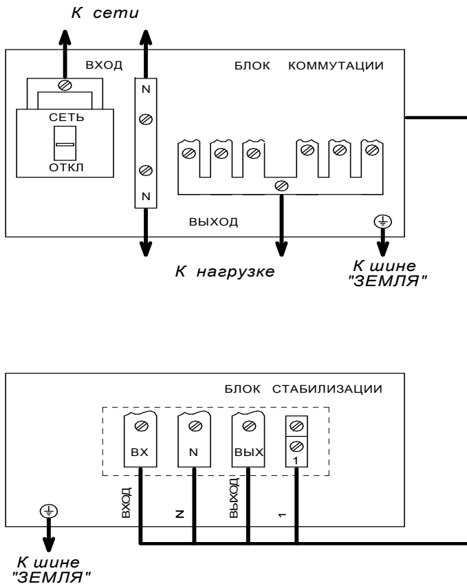
Рис. 6.1 Схема подключения изделия
